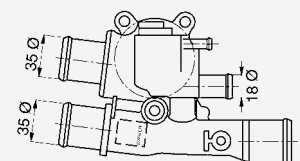
Typ 3163 mit M 12 x 1,5 3481 mit M 12 x 1,5 / M 16 x 1,5
