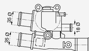
Typ 3163 mit M 12 x 1,5 3481 mit M 12 x 1,5 / M 16 x 1,5
