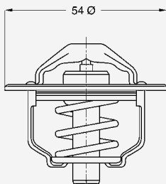
Typ 3116 mit Entlüftungsventil
