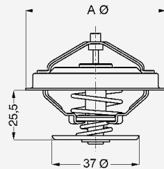
Typ A B 4049 67 37 ohne Entlüftungsventil oder -kerbe 4088 67 37 ohne Entlüftungsventil oder -kerbe 4132 75 43 mit Entlüftungskerbe 4116 67 37 Ventilteller gummi-beschichtet 4117 67 37 mit Entlüftungskerbe
