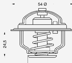
Typ 4003 ohne Entlüftungsventil oder -kerbe 4008 mit Entlüftungsventil 4015 mit Entlüftungsventil
