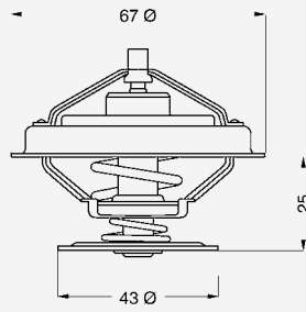
Typ 4165 mit Entlüftungsventil
