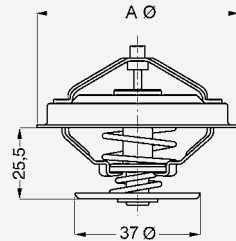
Typ A B 4049 67 37 ohne Entlüftungsventil oder -kerbe 4088 67 37 ohne Entlüftungsventil oder -kerbe 4132 75 43 mit Entlüftungskerbe 4116 67 37 Ventilteller gummi-beschichtet 4117 67 37 mit Entlüftungskerbe
