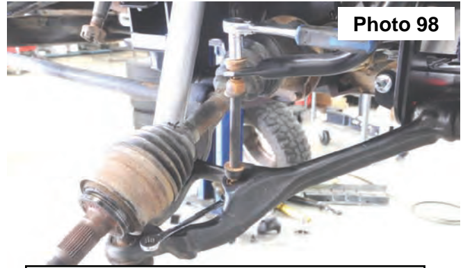
Tighten sway link bolt.
