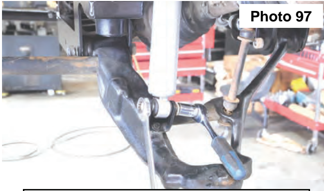
Install lower shock mount.
