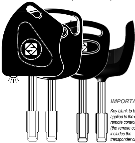
FO21T3L FO21T3 FO21P FO21AP FO21PL TIBBE (D) VALEO (F)
