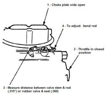
FIG. 11 - CHOKE UNLOADER
