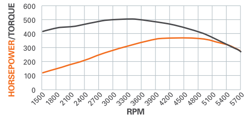
DYNO CHART
