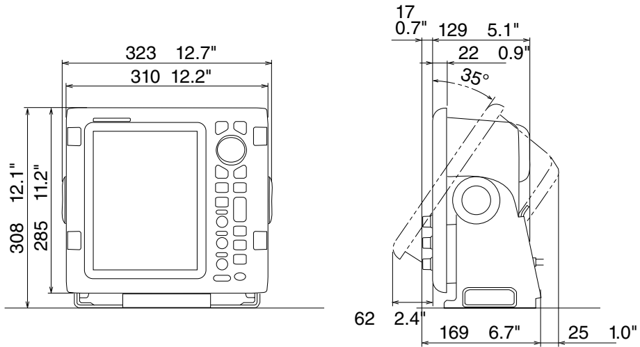
MODEL 1835/1935/1945 Display Unit
