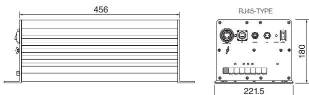
TRANSCIEVER
