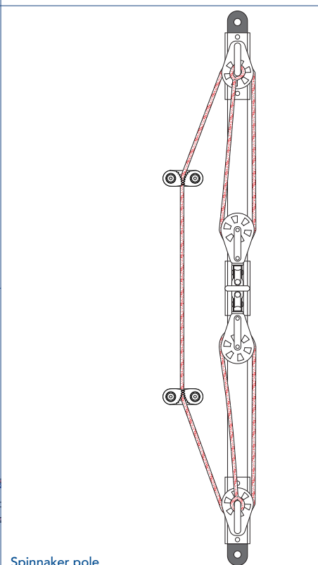
Spinnaker pole
