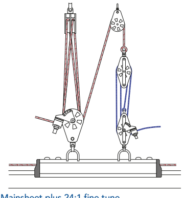
6:1 Mainsheet plus 24:1 fine tune
