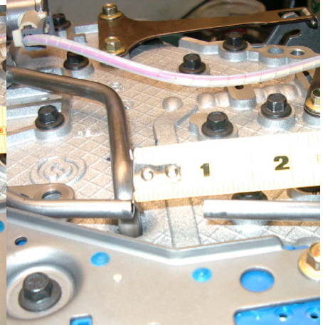
7/8" gap
