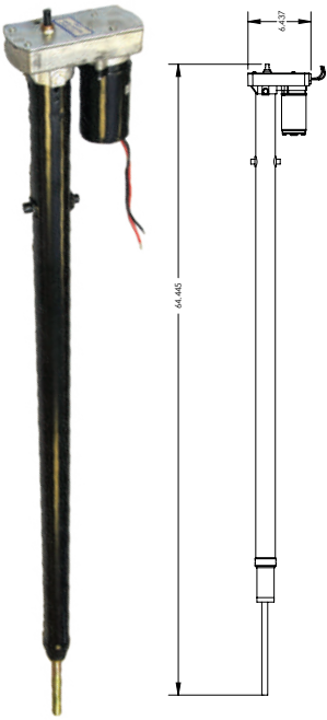
014-119129 - 40" Venture Actuator - 18:1 Motor
