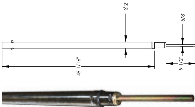
014-145595 - Venture Actuator
