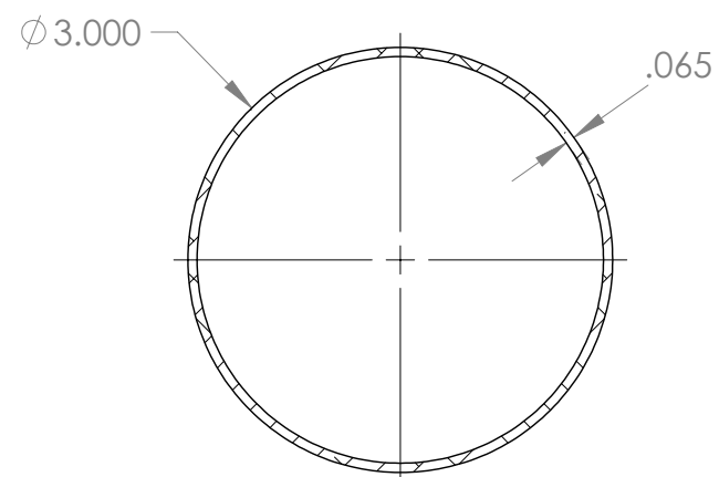
SECTION A-A SCALE 1 : 1.5
