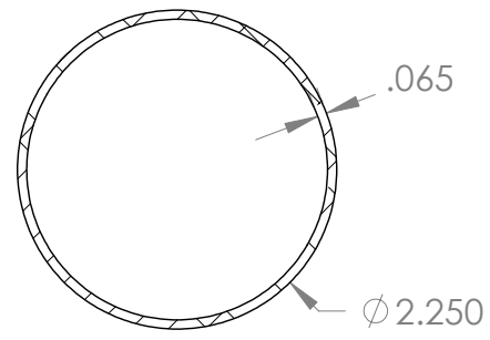
SECTION A-A SCALE 1 : 1.5
